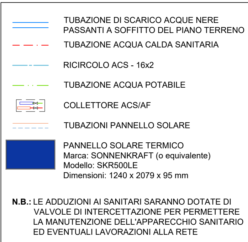
LEGENDA IMPIANTO IDROSANITARIO
