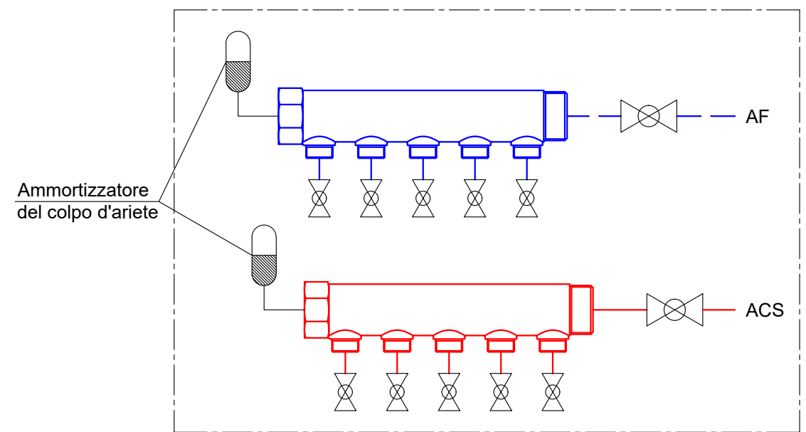
SCHEMA ALLACCIAMENTI NUOVI COLLETTORI DI DISTRIBUZIONE LAVABI-DOCCE-VASI
