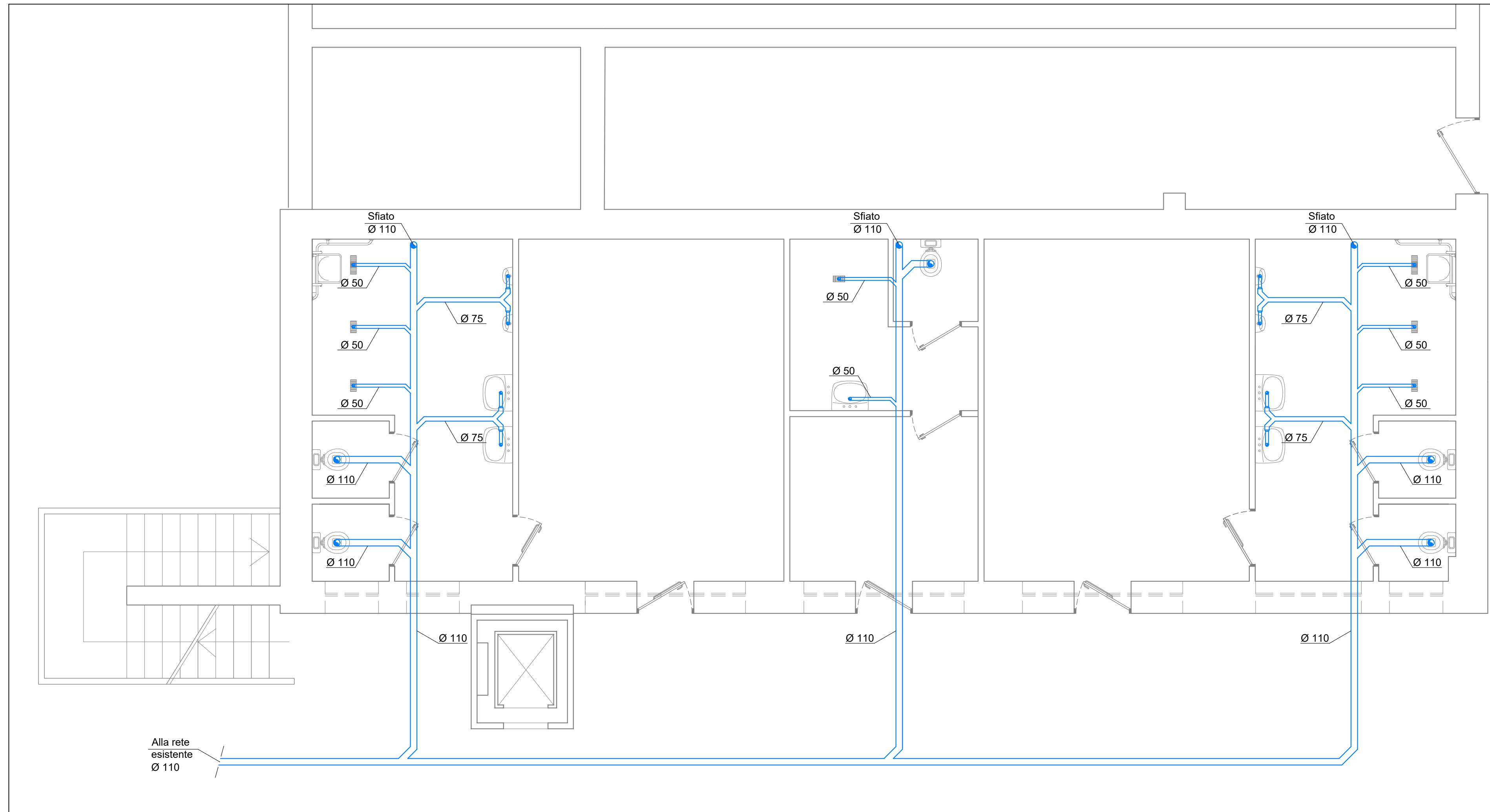
SERVIZIO IGIENICO - SCARICHI - SCALA 1:50
